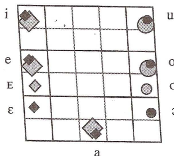
Fig.2. Quadrilatero vocalico 2
